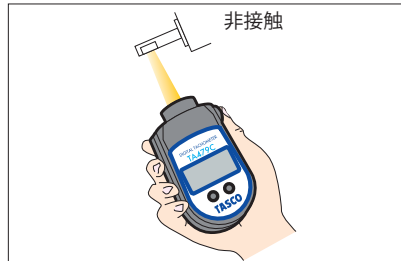
■ 本機からの光を、被測定物に張りつけた反射テープに照射します。
